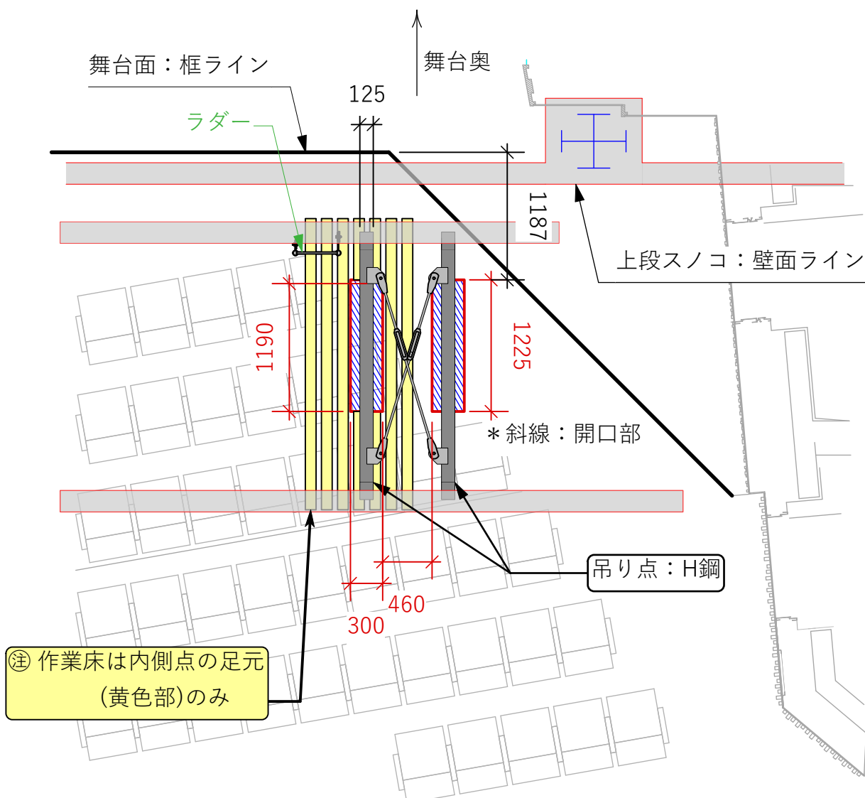
平面図 (上手側)
